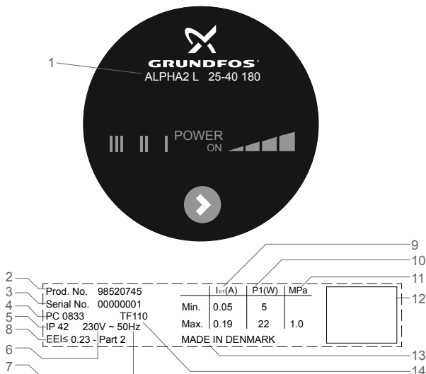
2-сур. ALPHA2 L фирмалық тақтасының мысалы
