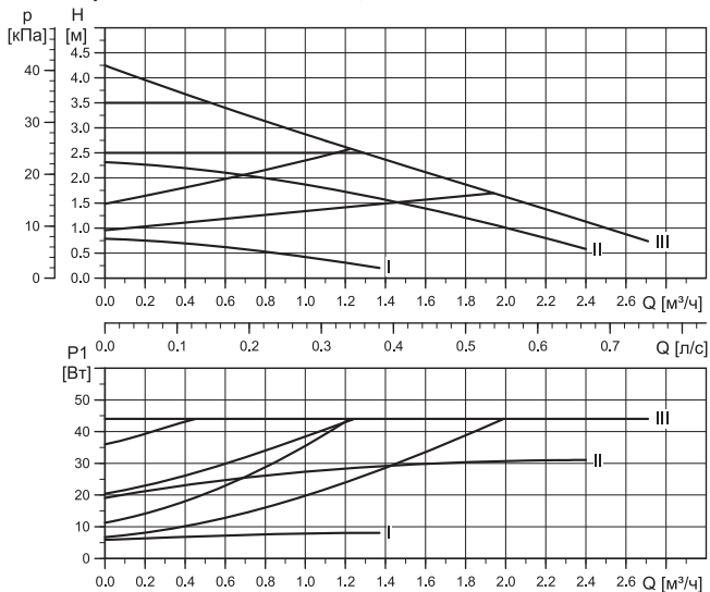
18-сұр. ALPHA2 L XX-45
