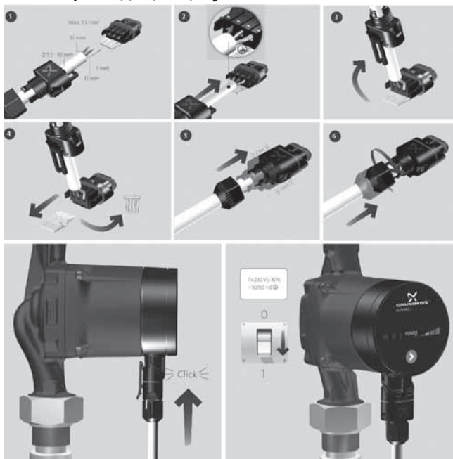
7-сур. Электр құрылғысын іске қосу
