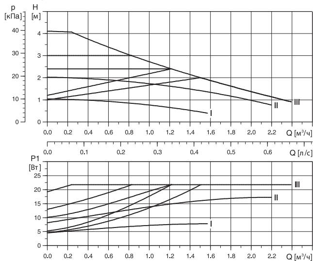
17-сұр. ALPHA2 L XX-40
