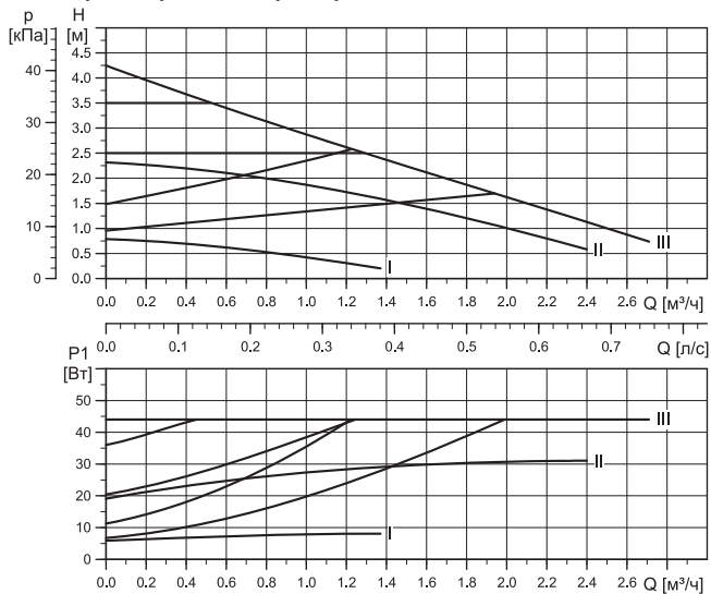
Рис. 18 ALPHA2 L XX-45
