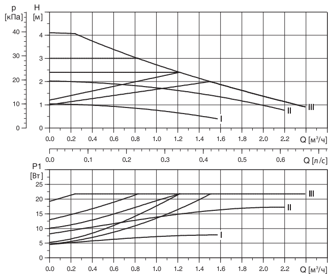
Рис. 17 ALPHA2 L XX-40
